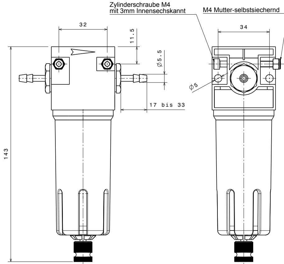
Vorderansicht
