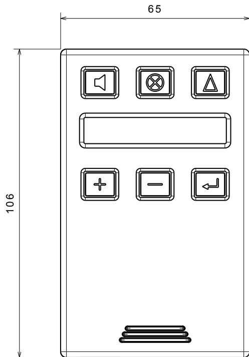
Vorderansicht
